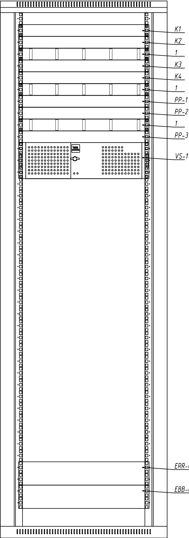
Вид спереди
