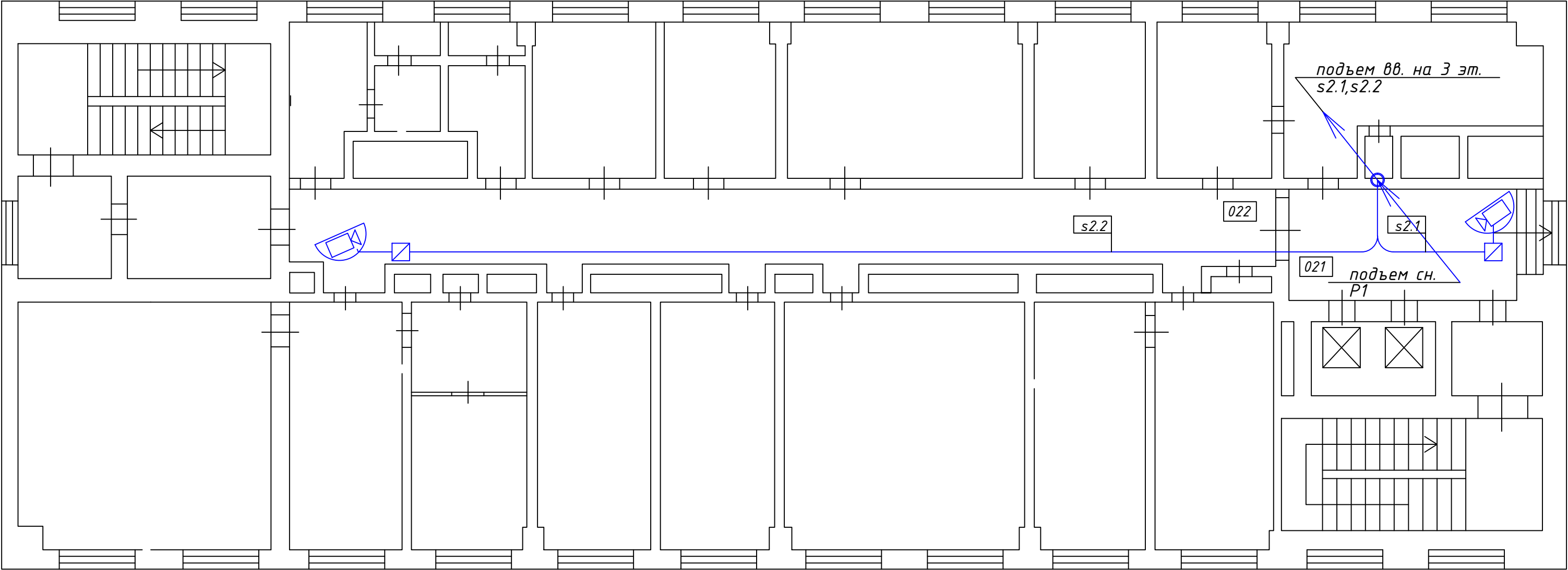
План 2 этажа
