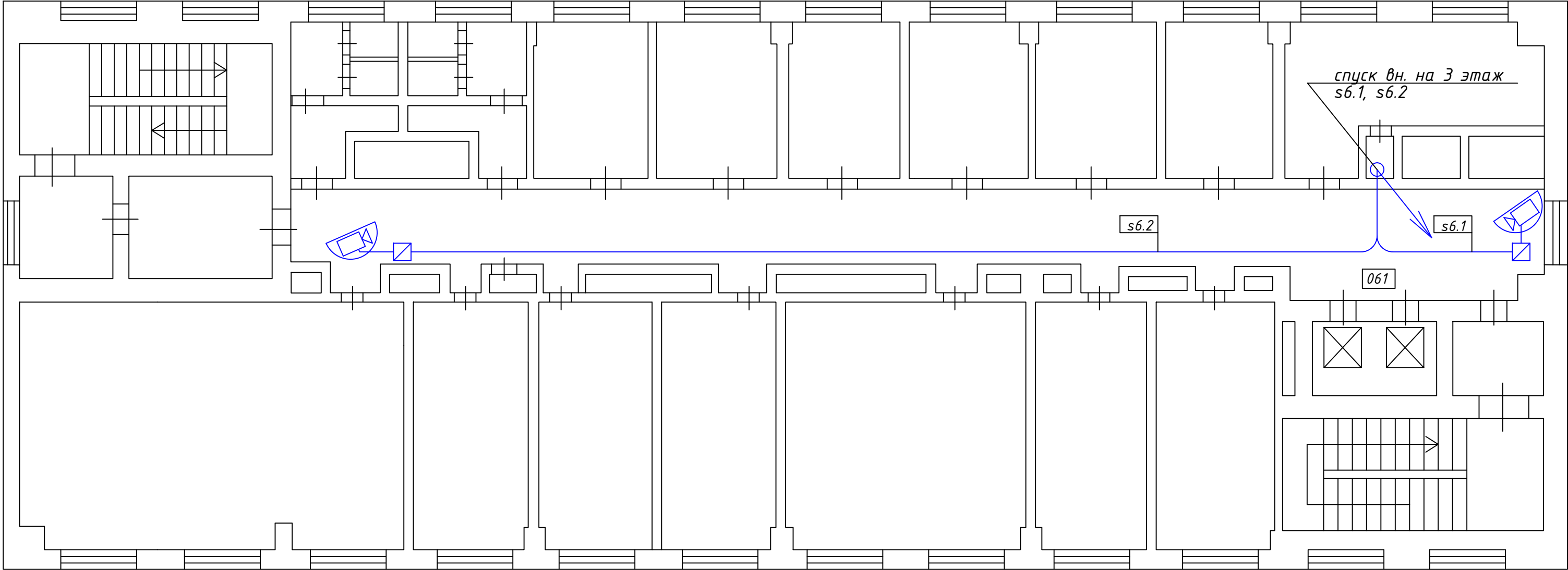
План 6 этажа
