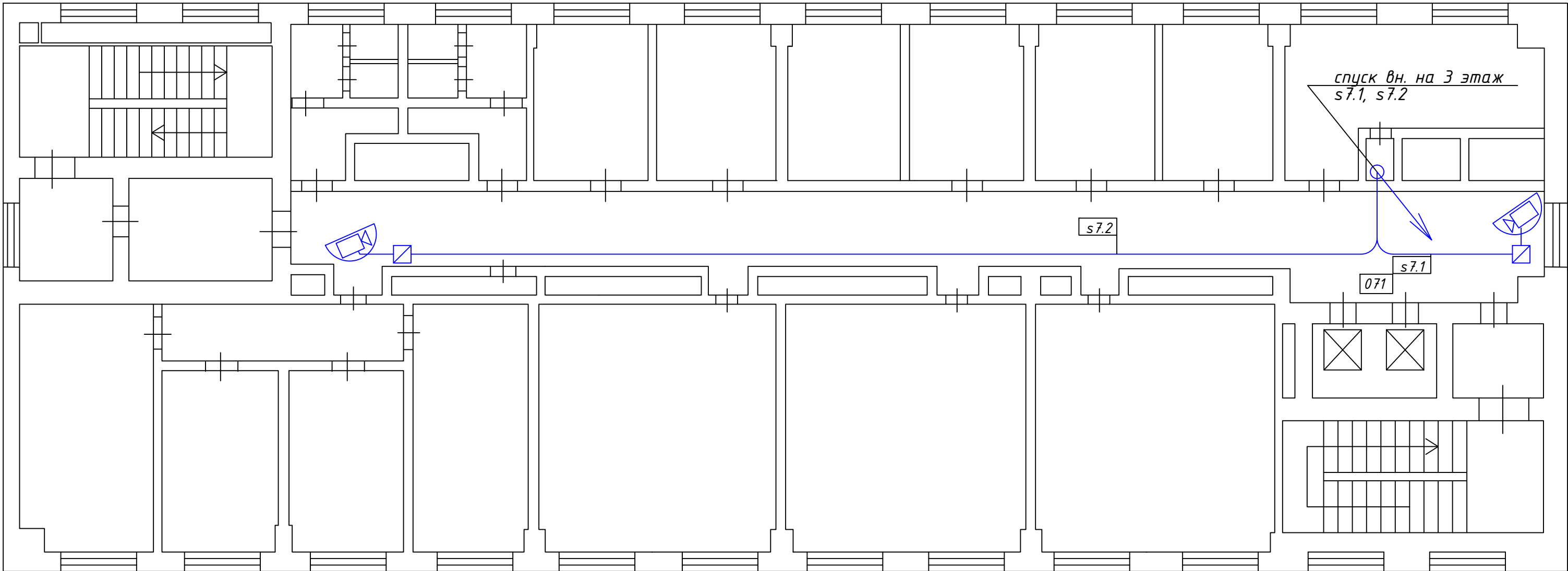
План 7 этажа
