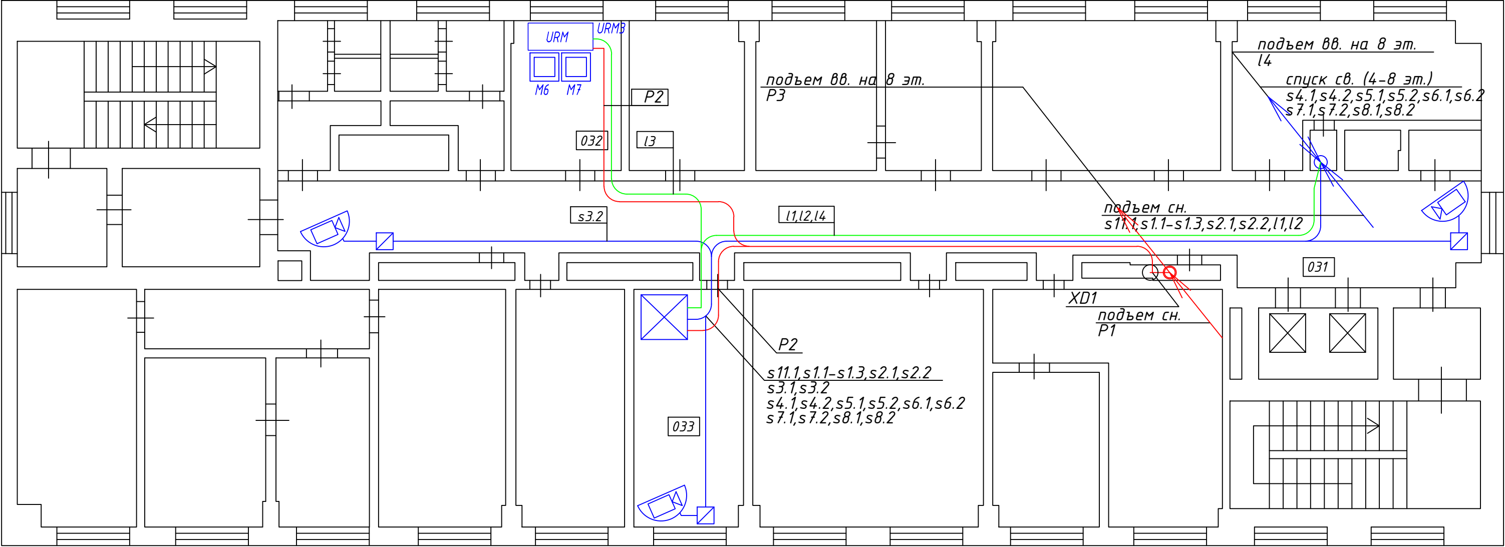
План 3 этажа
