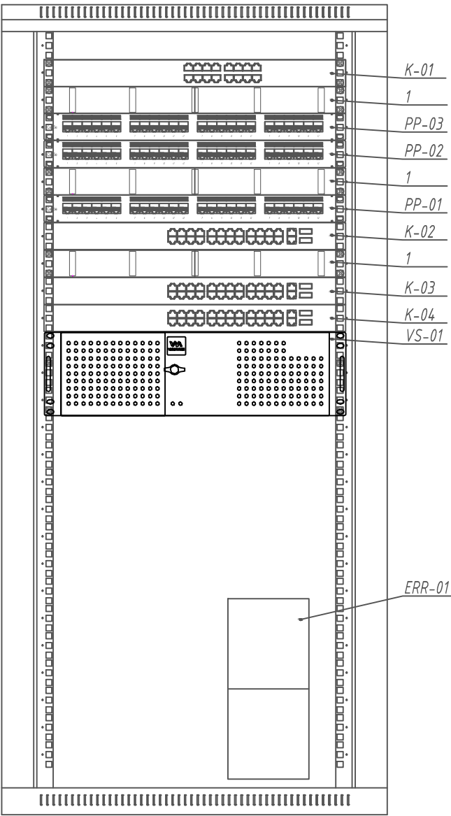
Вид спереди
