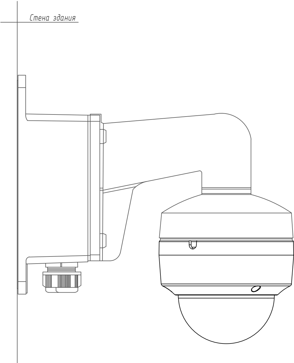
Крепление купольной сетевой видеокамеры в термокожухе DS-2CD2122FWD-I на стену (схема для внешней установки)
