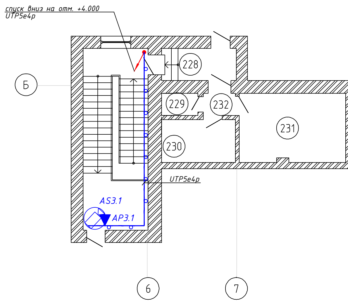
План 3-го этажа на отм. + 5.530
