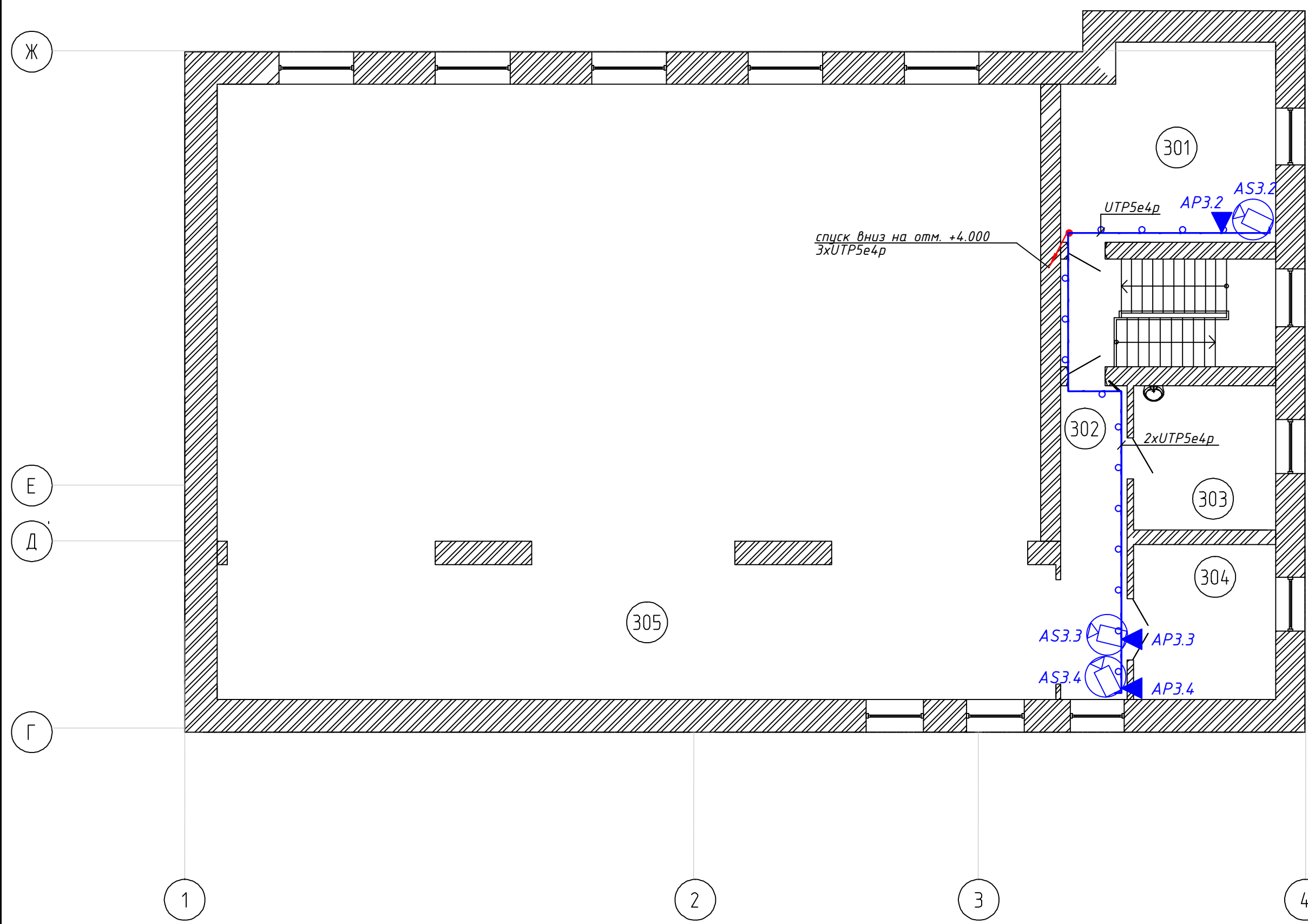
План 3-го этажа на отм. + 5.730
