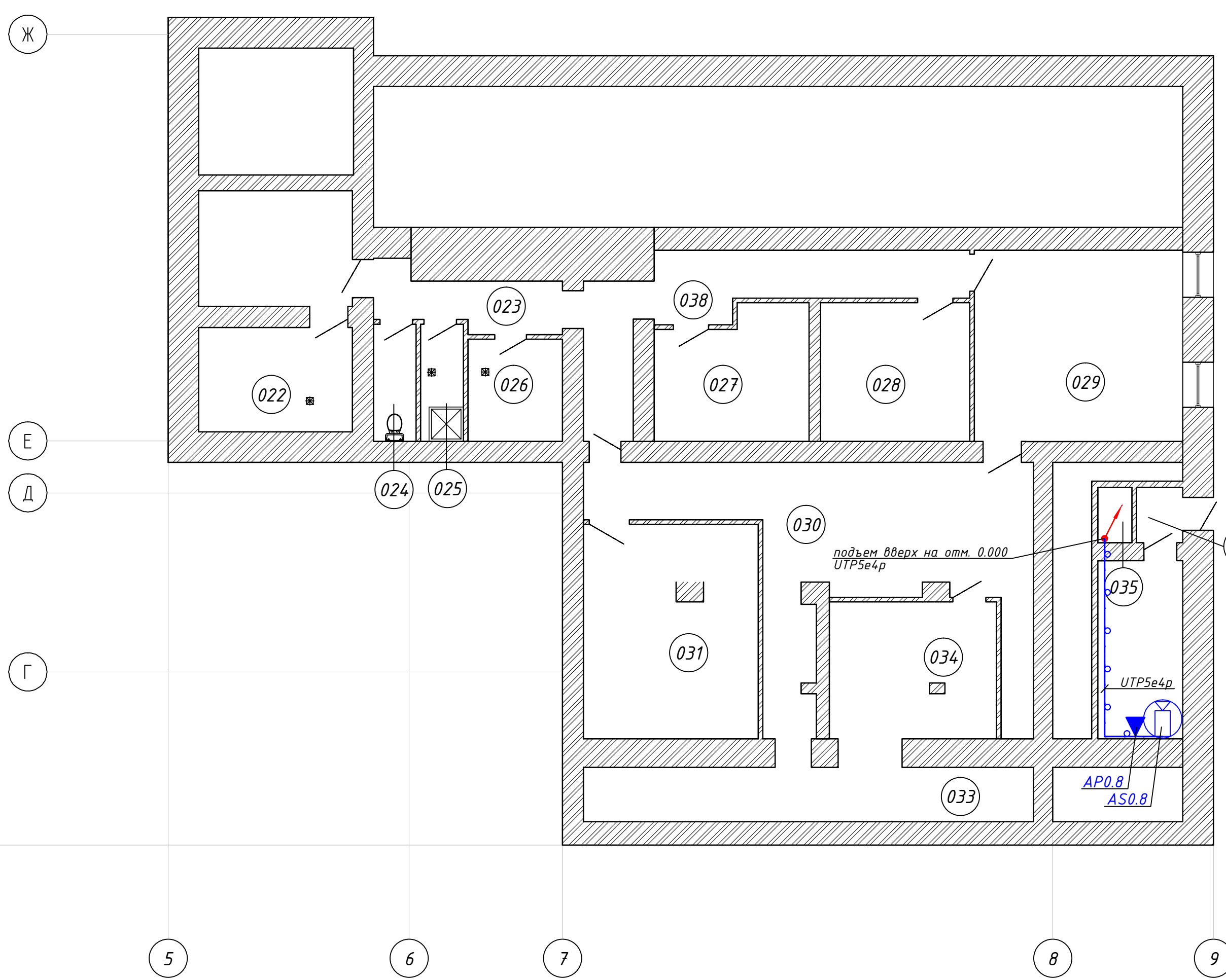
План подвала
