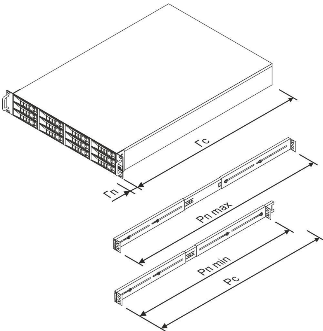
Рис. 7 Исходные геометрические данные для подбора Шкафа.
