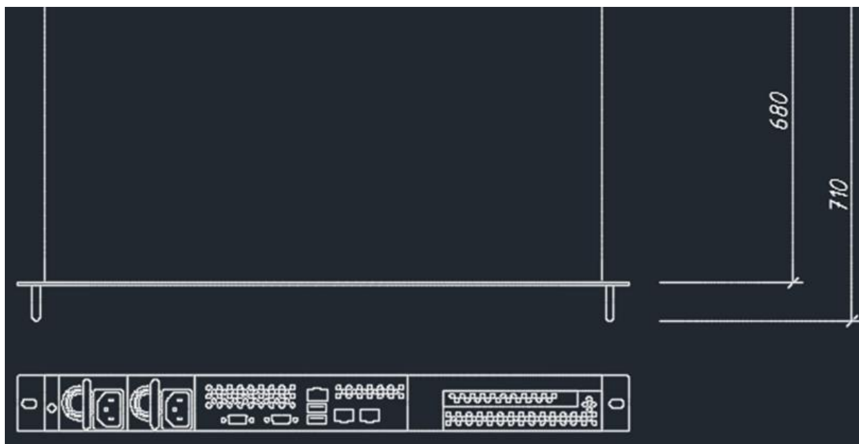
Рис. 9 Габариты Сервера в DWG-файле.
