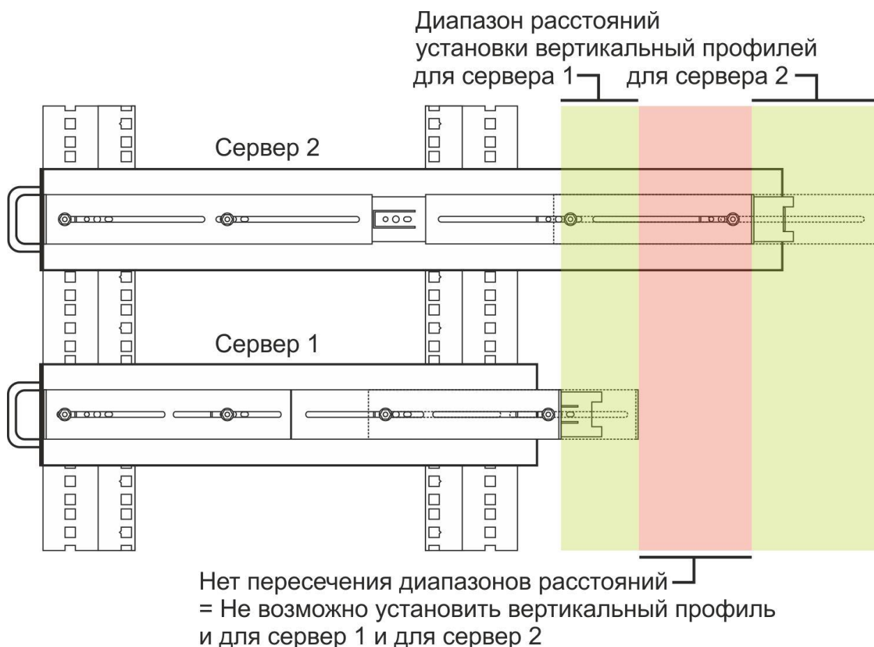
Рис. 11 Пример отсутствия «пересечения» салазок.
