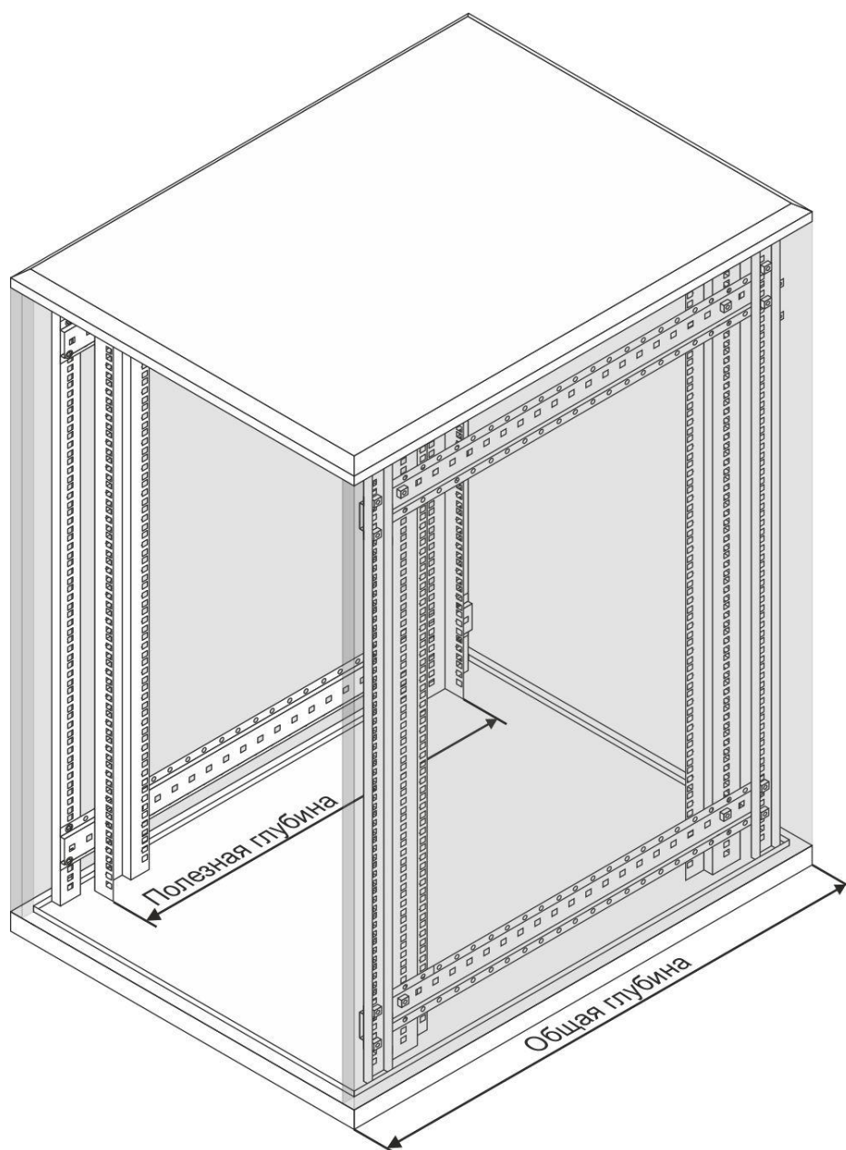
Рис. 1 Общая и полезная глубины Шкафа.
